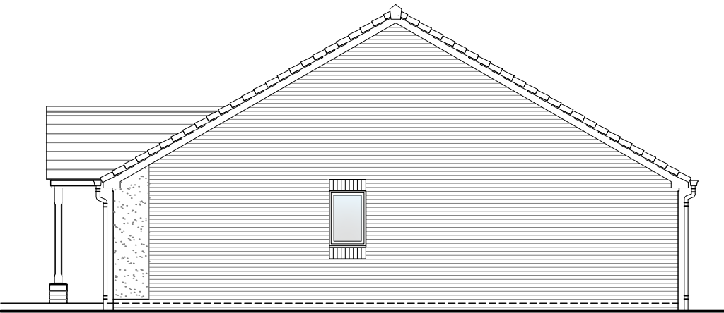
Right Elevation
